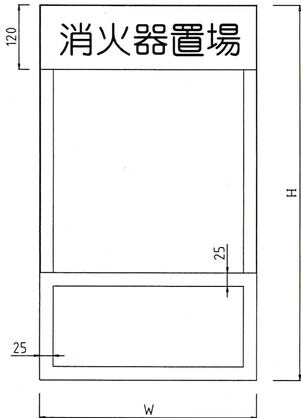
正面図
