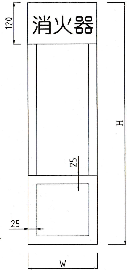
正面図
