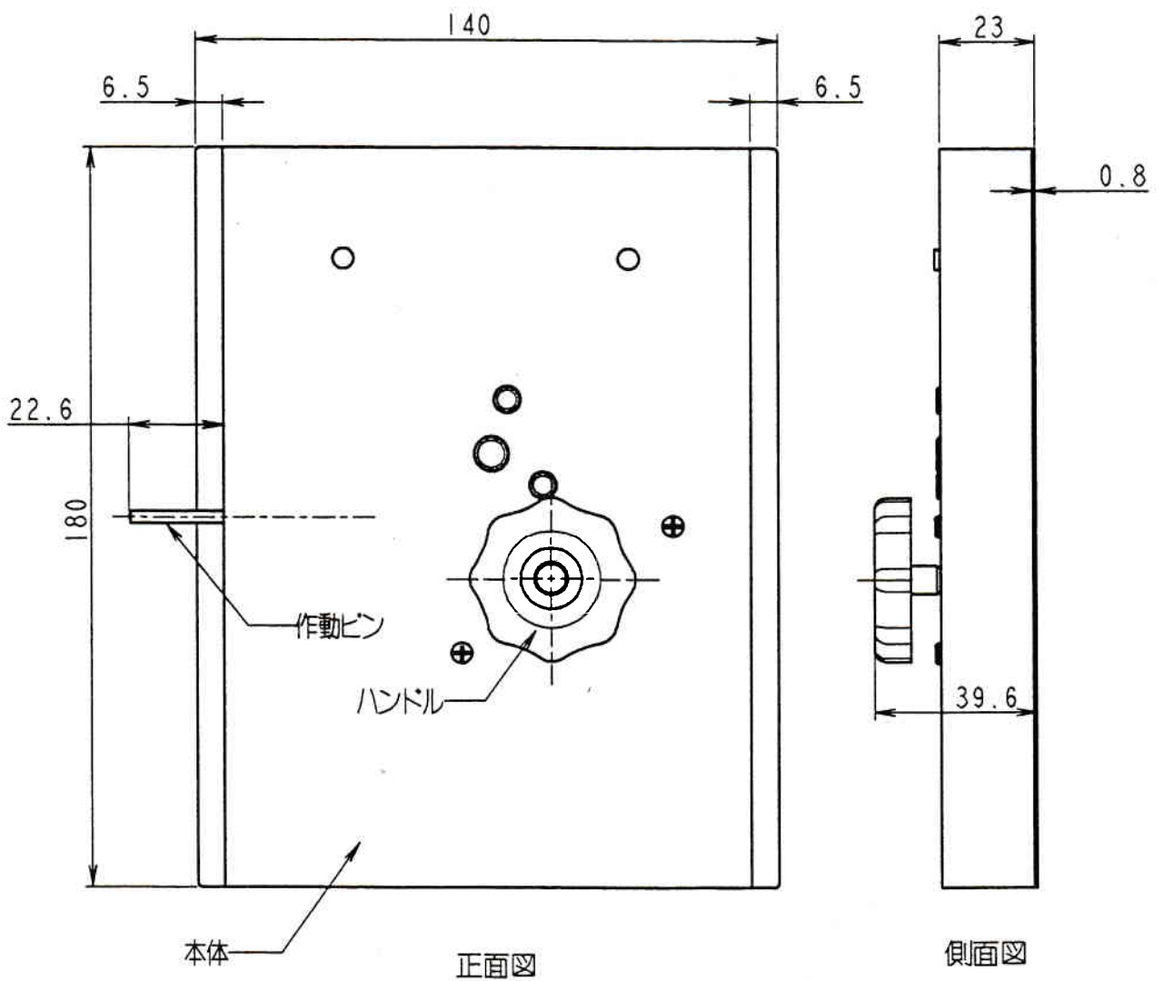
図3 角ベル概略図 (単位: mm)
