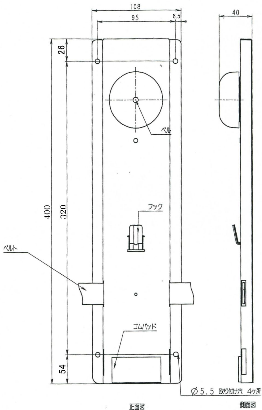
図3 ブラケットベル(L) 概略図 (単位:mm)
