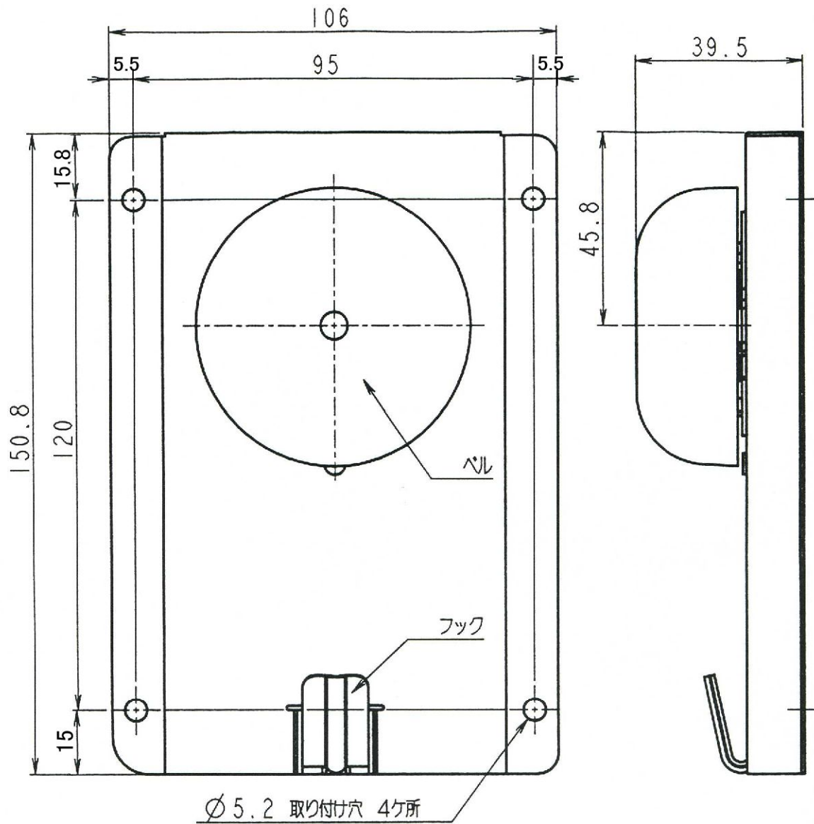
側面図
